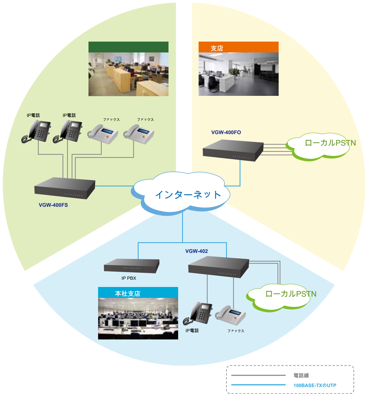
4ポートSIPゲートウェイ ( VGW-400FO )
